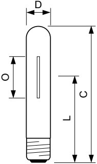
SON GreenPower CG T 250W E40
